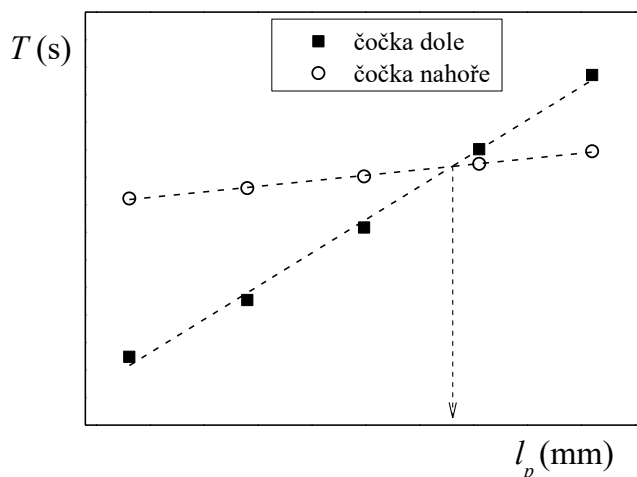
Obr. 3. Grafická interpolace
